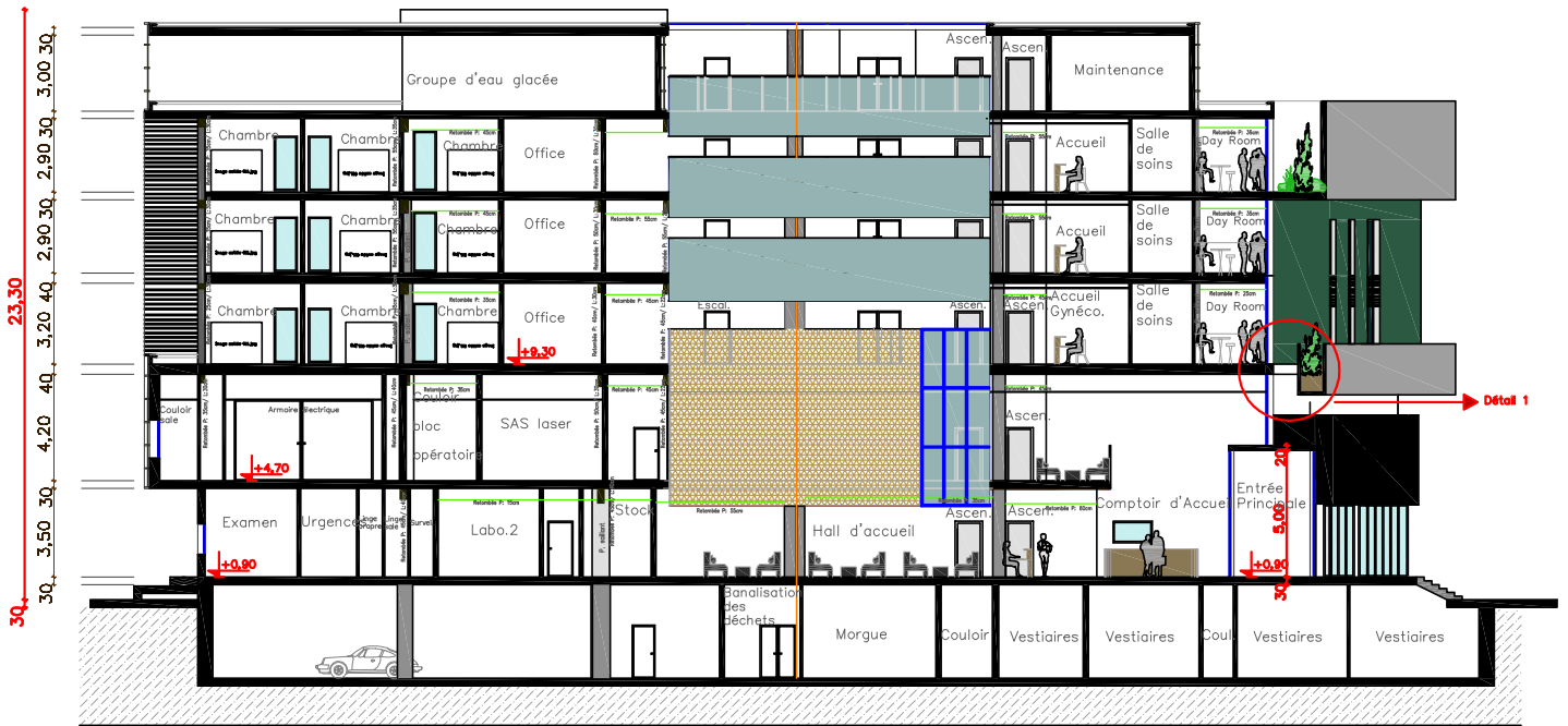
Coupe B-B
